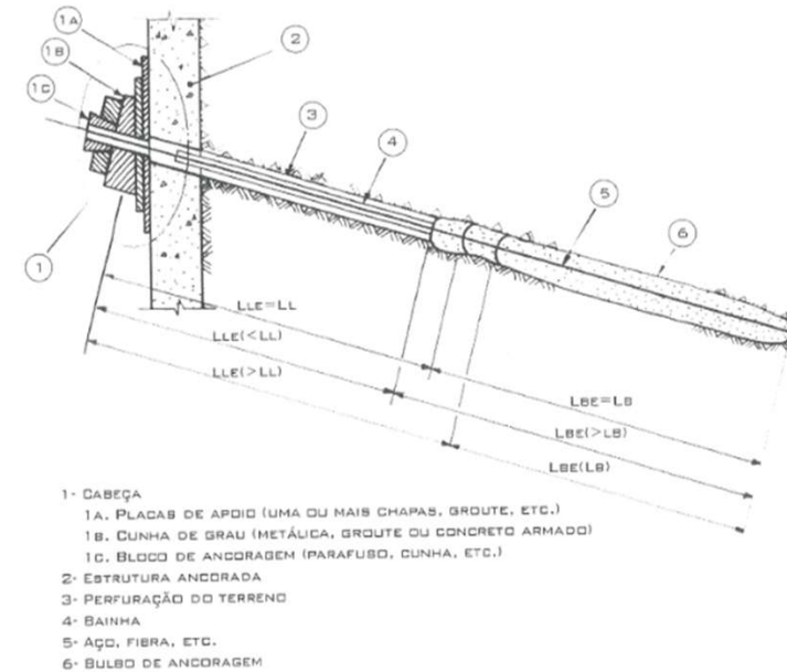
ELEMENTOS DO TIRANTE
