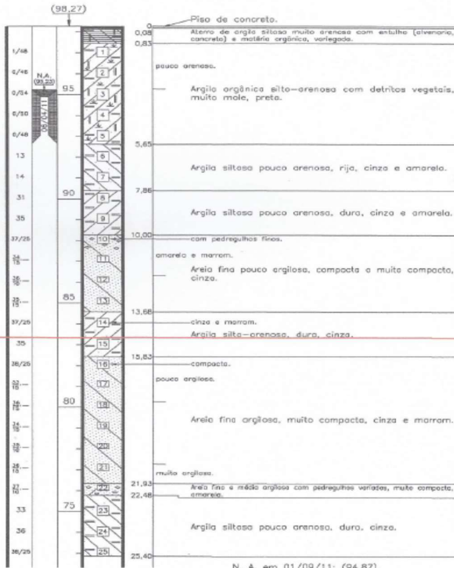
SONDAGEM SP-2
