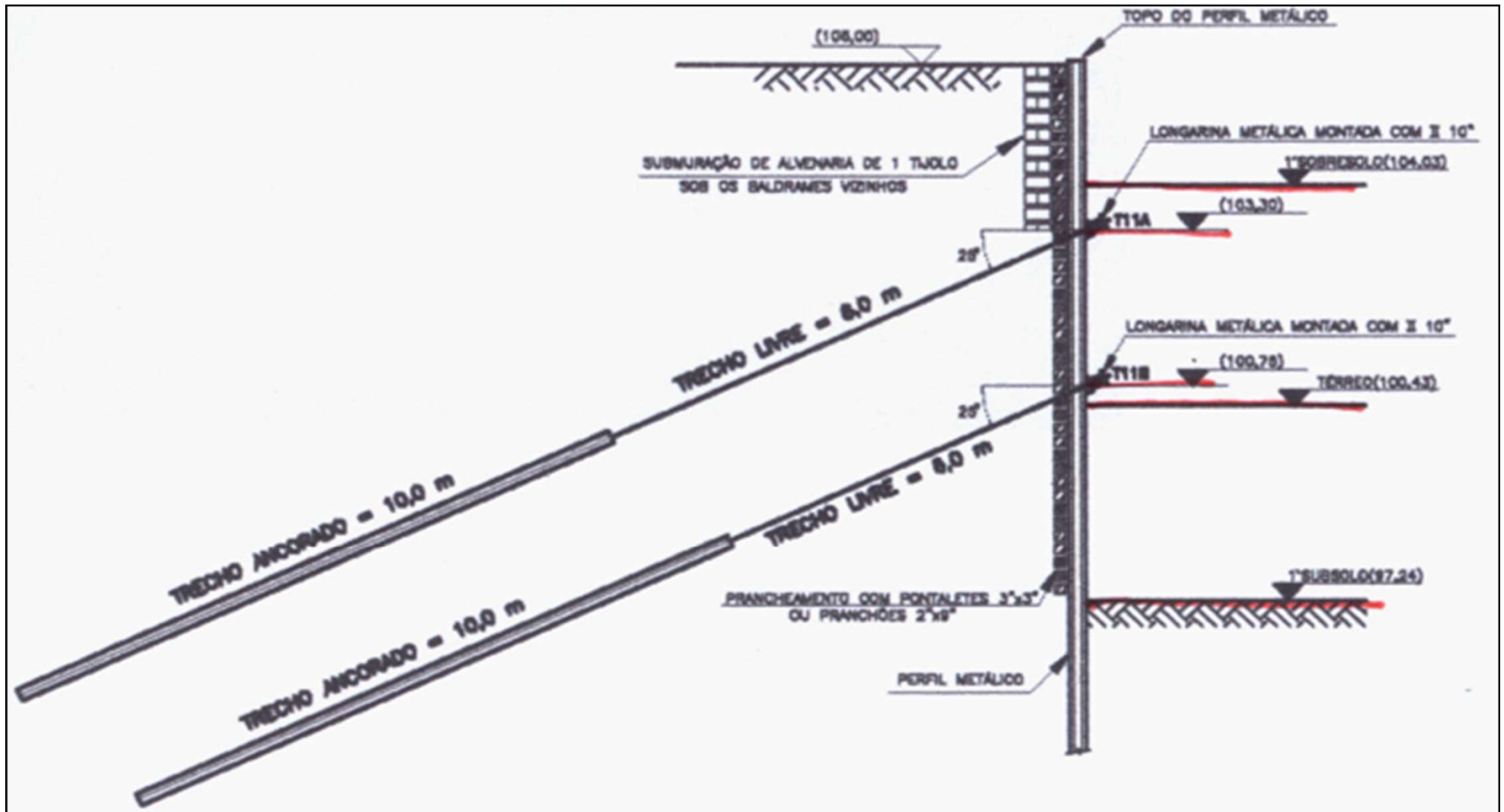
Corte B-B
