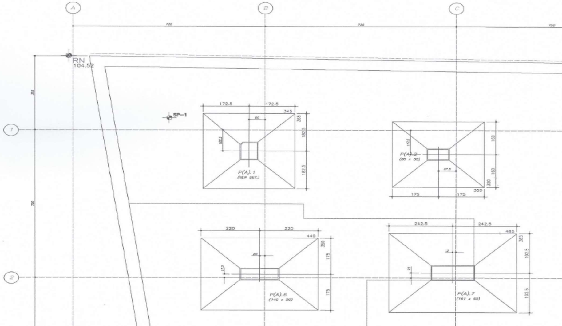
TRECHO DO PROJETO DAS SAPATAS
