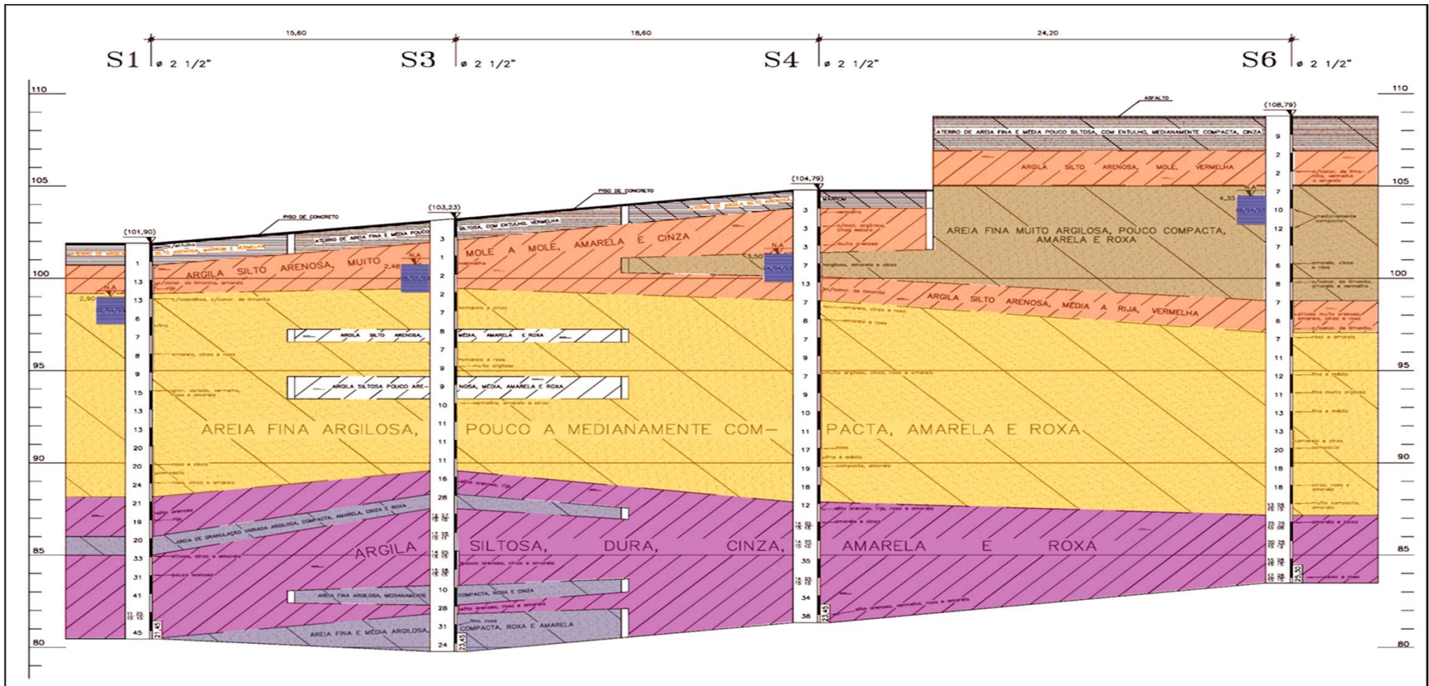
Secção do subsolo – S1, S3, S4, S6
