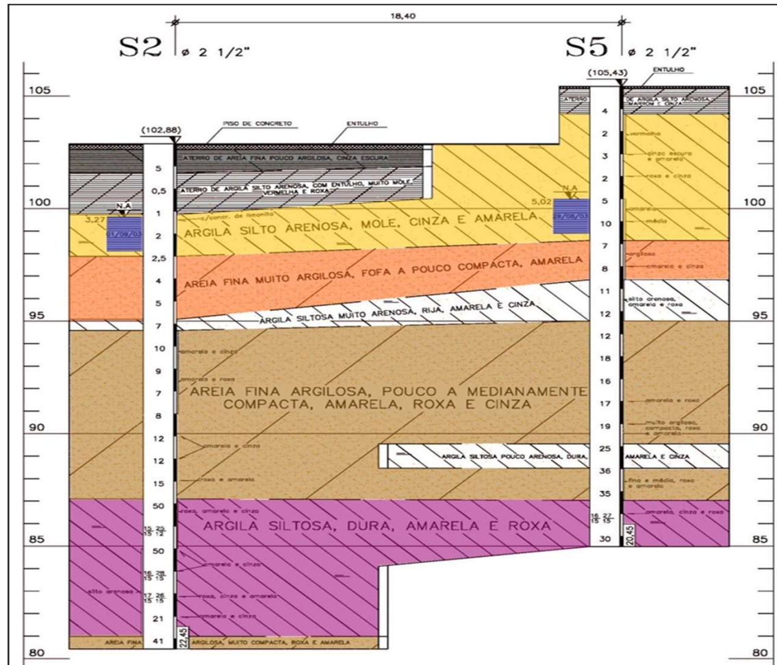
Secção do subsolo – S2 e S5
