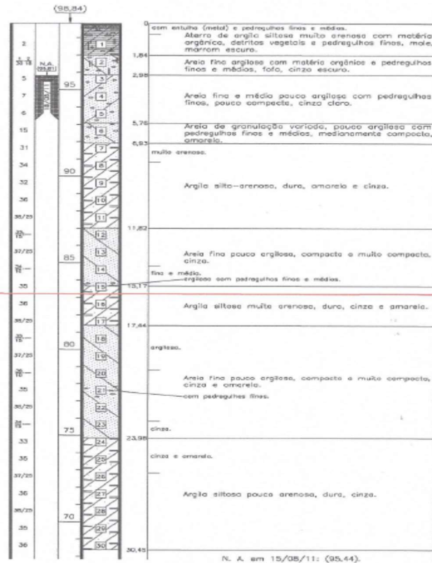
SONDAGEM SP-7
