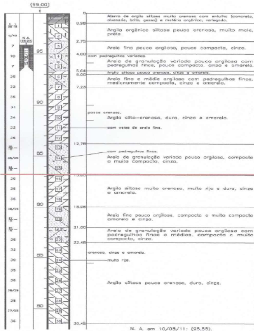
SONDAGEM SP-8
