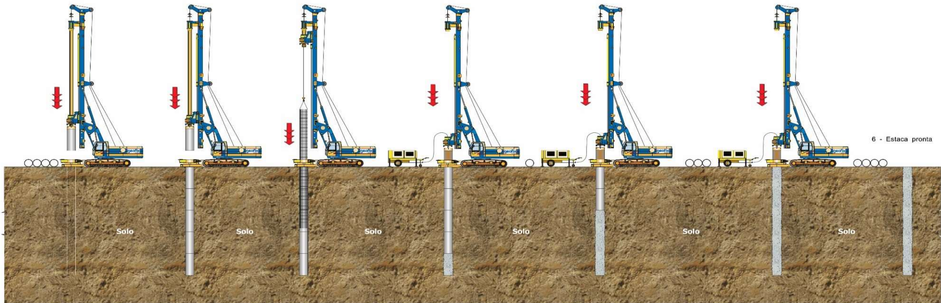
4 - Retirada de tubos com complemento de argamassa
