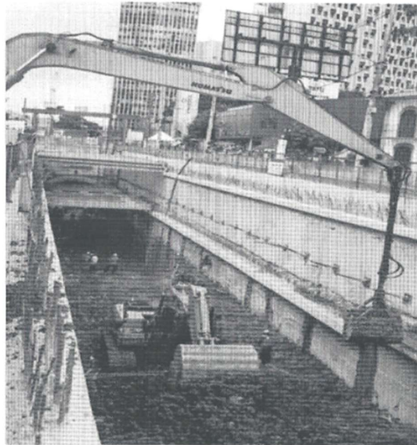
Túnel da Av. Cidade Jardim
