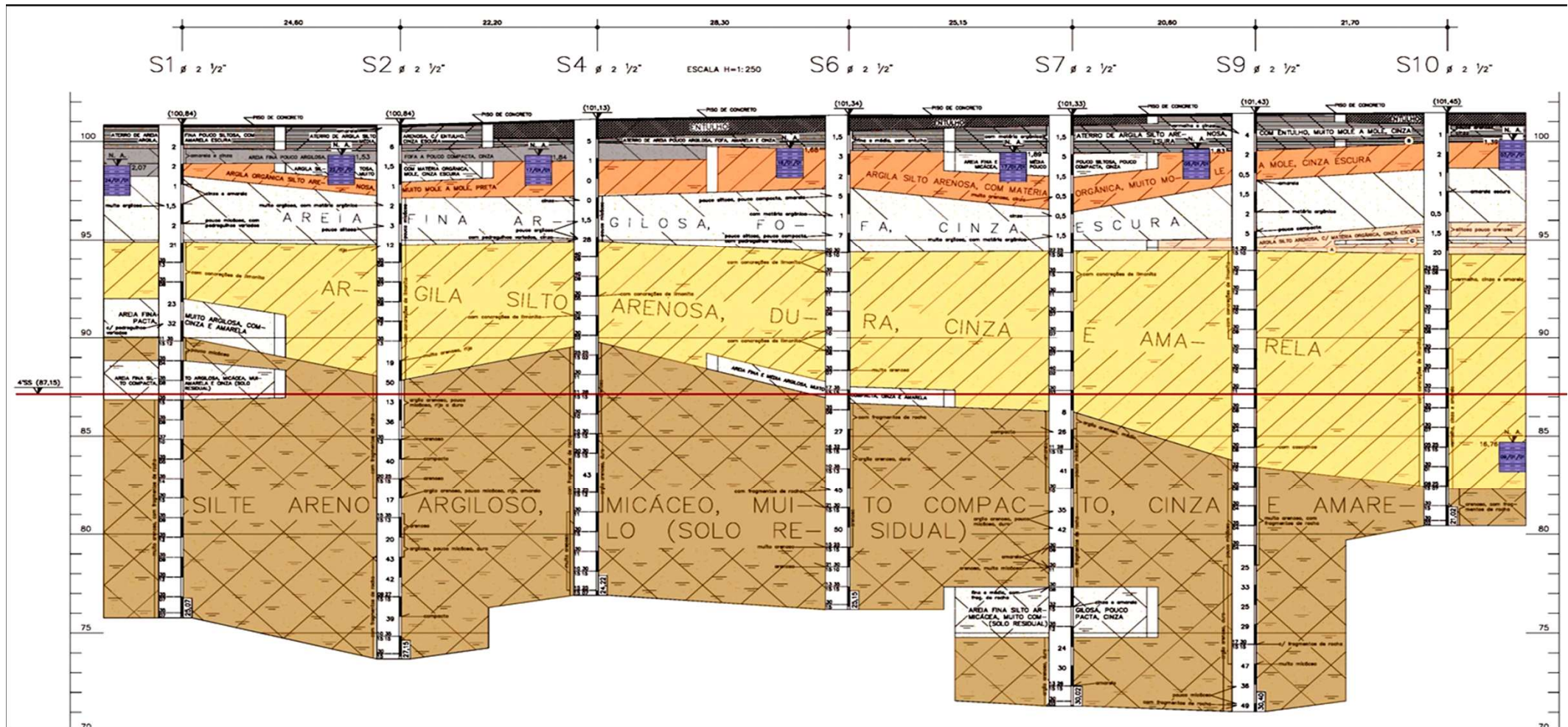
Secção do subsolo – S1, S2, S4, S6, S7, S8, S9, S10
