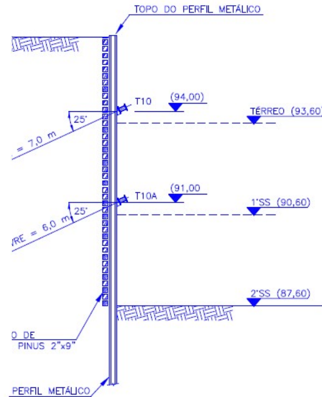
CORTE A-A
