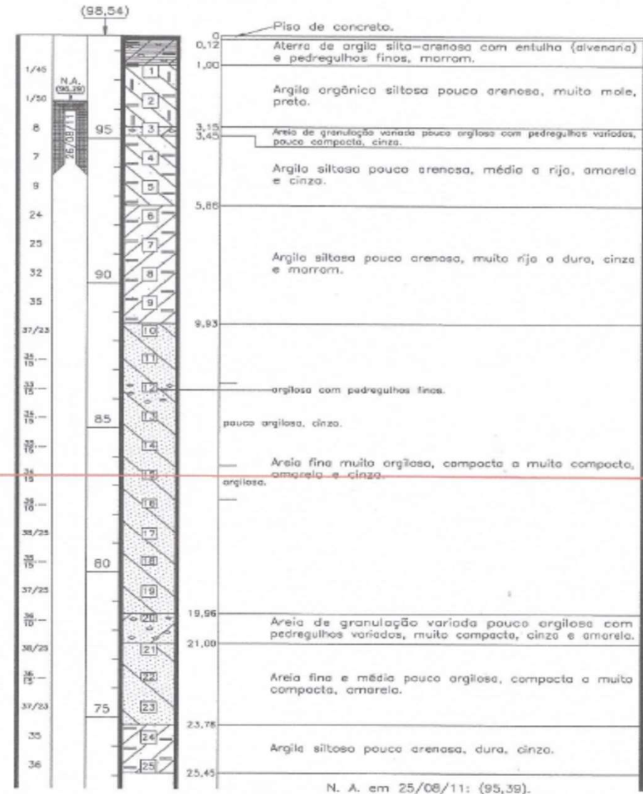
SONDAGEM SP-1
